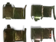
1 KI 13 Alinhador de pastilha
