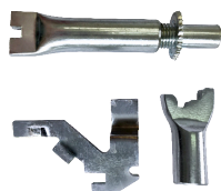
4 GM 68D Regulador de freio
